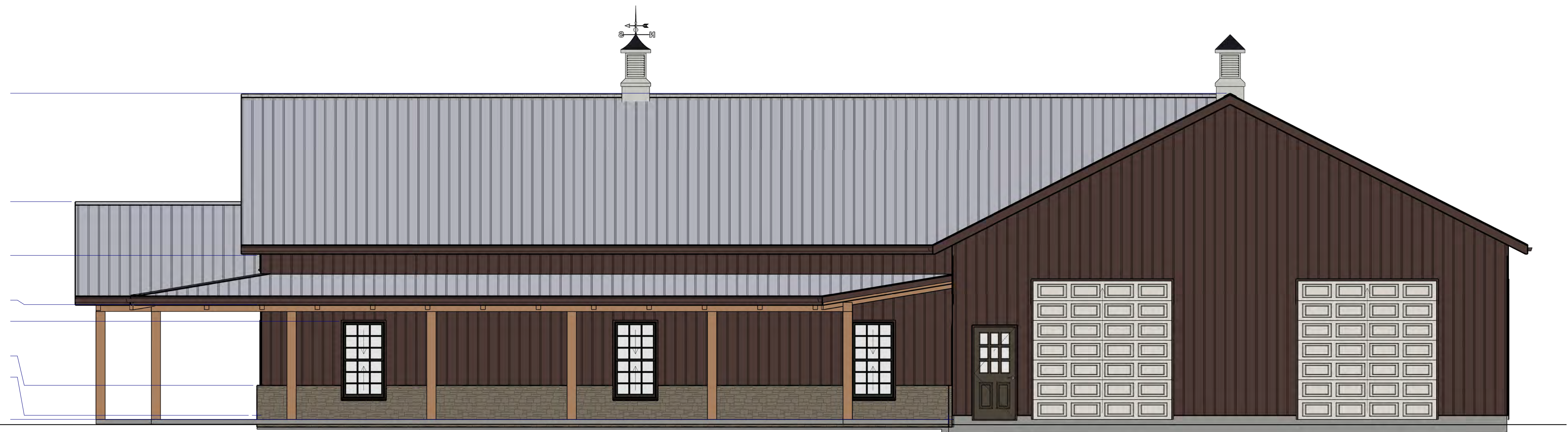
E4 Right Elevation
